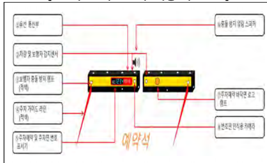
[ 스마트 카스토퍼 기능 구조도 ]
